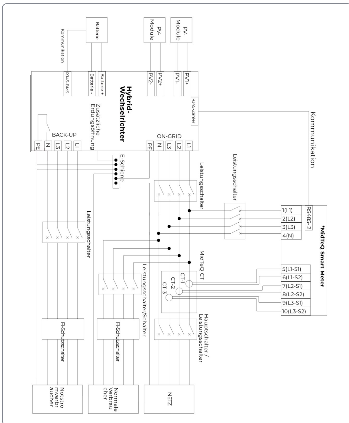
Abbildung 5-3 einfacher Schaltplan
