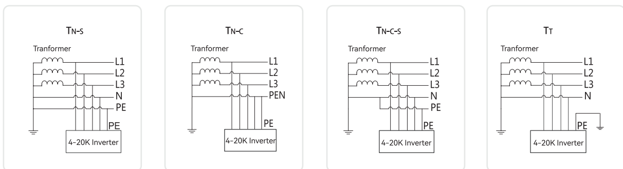
Abbildung 3-2 Anwendbare Stromnetztypen
