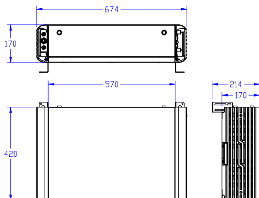
Battery module
