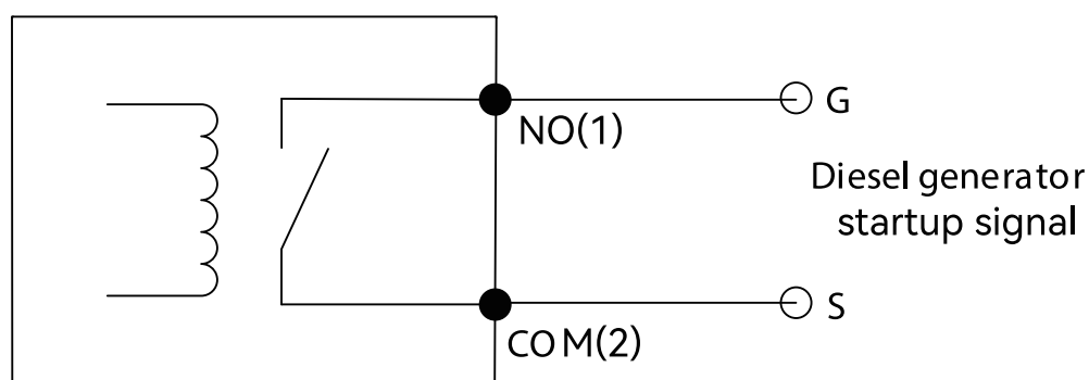
Abbildung 5-26 Anschlussschema Generatorsteuerung
