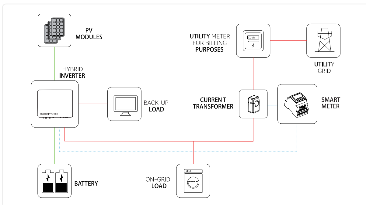
Abbildung 3-1 Schematische Darstellung des Hybridsystems
