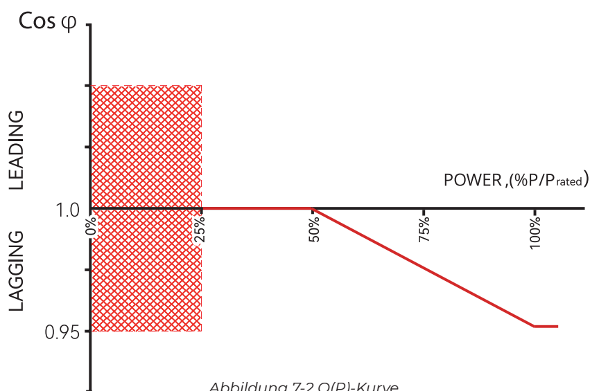
Abbildung 7-2 Q(P)-Kurve
